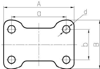
平底固定底板 Plate of Rigid Caster
