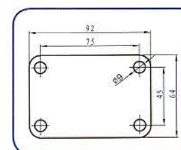
活动底板 Swivel baseplate
