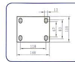
5"、6"、8" 底板 5"、6"、8" Baseplate
