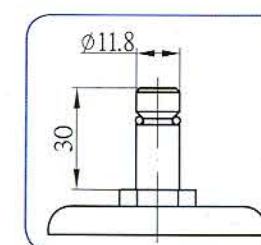
插杆 stem
