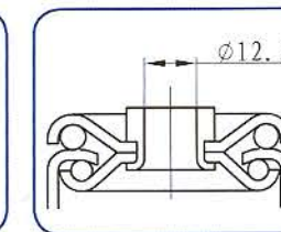
顶孔 Bolt hole
