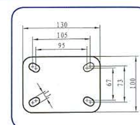
3.5-5 寸活动底板 3.5-5" Swivel baseplate
