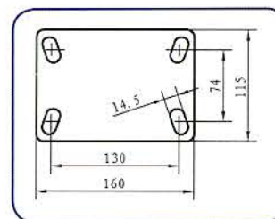
6"、8"底板 6"、8" Baseplate
