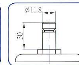
插杆 stem
