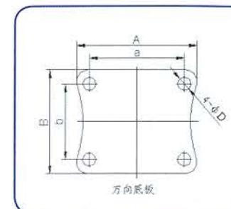
1"-3" 活动底板图 1"-3" Swivel baseplate
