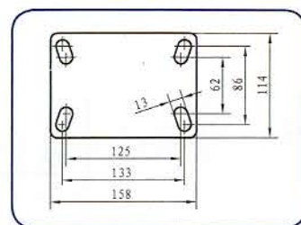
底板 Baseplate
