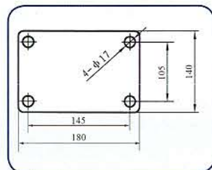
10" 底板 10" Baseplate
