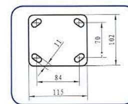
底板 Baseplate
