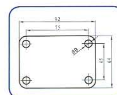
活动底板 Swivel baseplate
