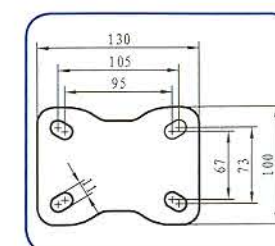
3.5-5 寸固定底板 3.5-5" Rigid baseplate
