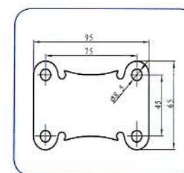
固定底板 Rigid baseplate
