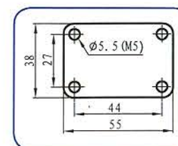
1.5寸底板 1.5" Baseplate
