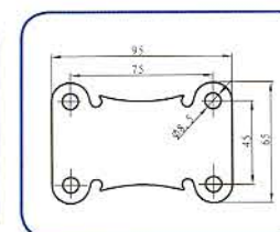
固定底板 Rigid baseplate
