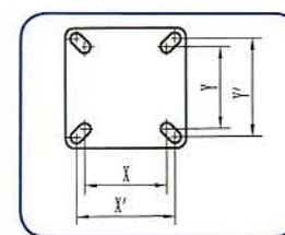
活动底板 swivel baseplate
