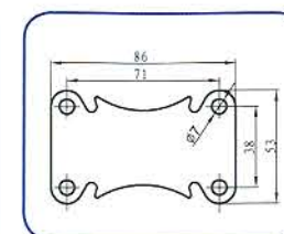
2-2.5寸固定底板 2-2.5" Rigid baseplate
