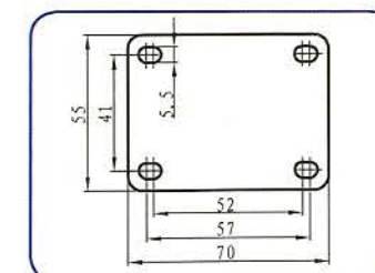
底板 Baseplate
