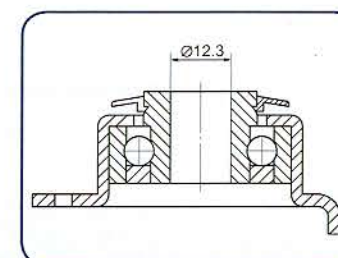
顶孔 Bolt hole
