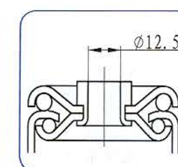
顶孔 Bolt hole
