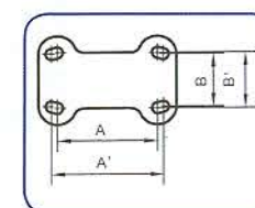
固定底板 rigid baseplate
