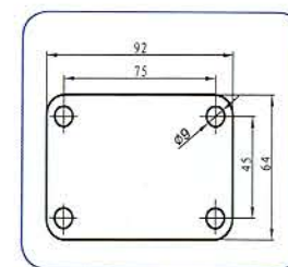
活动底板 Swivel baseplate
