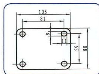
底板 baseplate
