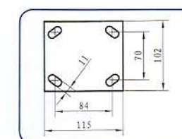
底板 Baseplate
