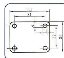
2-3 寸底板 2-3" baseplate
