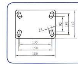
10"、12" 底板 10"、12" Baseplate
