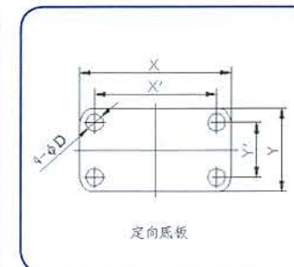
1"-3" 固定底板图 1"-3" Rigid baseplate
