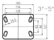
平底固定底板 Plate of Rigid Caster
