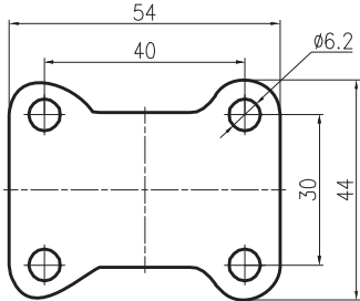
平底固定底板 Plate of Rigid Caster
