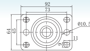
平底活动 刹车底板 Plate of Swivel Caster
