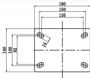
平底活动 刹车 / 固定底板 Plate of Swivel / Rigid Caster
