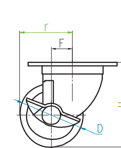
平底活动 刹车底板 Plate of Swivel Caster
