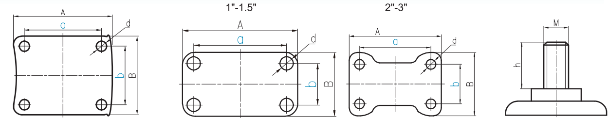
平底活动 刹车底板 Plate of Swivel Caster
