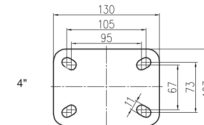
平底活动 刹车底板 Plate of Swivel Caster
