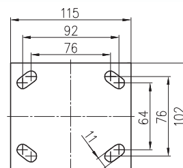
平底活动 / 固定底板 Plate of Swivel / Rigid Caster
