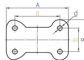
平底固定底板 Plate of Rigid Caster
