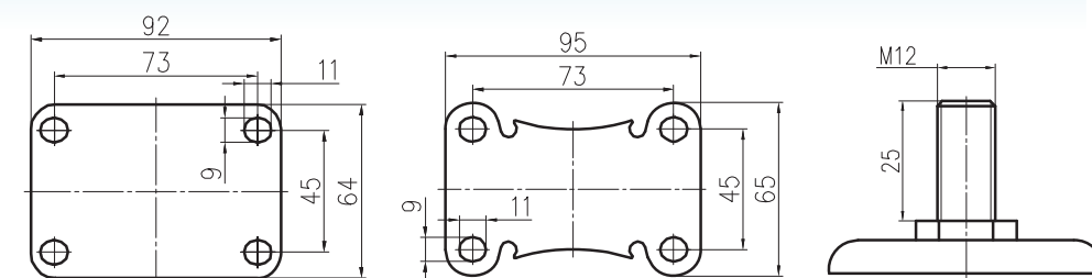
平底活动 刹车底板 Plate of Swivel Caster
