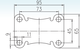
平底固定底板 Plate of Rigid Caster
