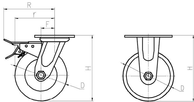
可选拉环刹 Optional Pull Ring Brake
