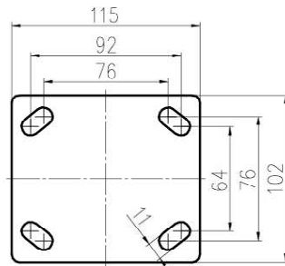
平底活动 刹车 / 固定底板 Plate of Swivel / Rigid Caster
