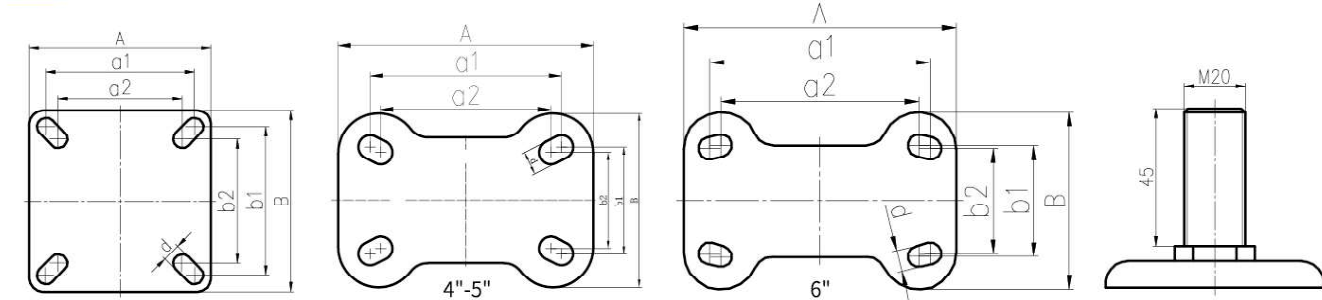
平底活动/ 刹车底板 Plate of Swivel Caster
