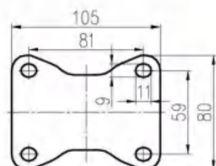
平底固定底板 Plate of Rigid Caster
