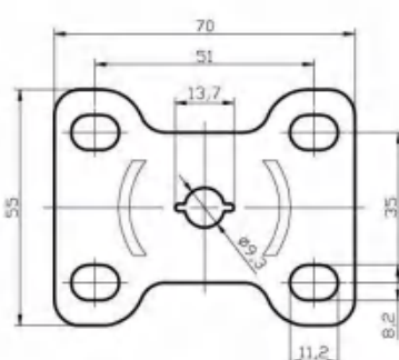
平底固定底板 Plate of Rigid Caster
