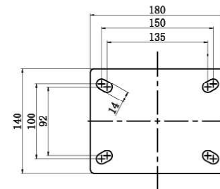
安装尺寸 Installation Drawing
