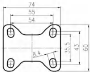
平底固定底板 Plate of Rigid Caster
