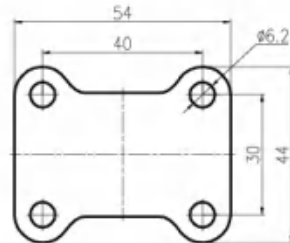
平底固定底板 Plate of Rigid Caster
