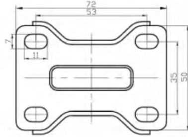
平底固定底板 Plate of Rigid Caster
