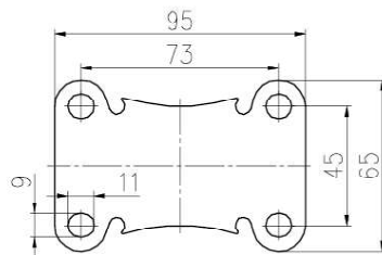
平底固定底板 Plate of Rigid Caster
