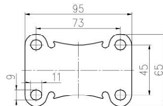
平底固定底板 Plate of Rigid Caster
