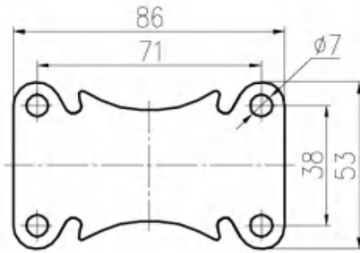
平底固定底板 Plate of Rigid Caster
