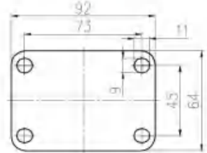
平底活动/ 刹车底板 Plate of Swivel Caster
