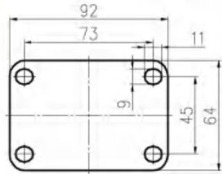
平底活动 刹车底板 Plate of Swivel Caster
