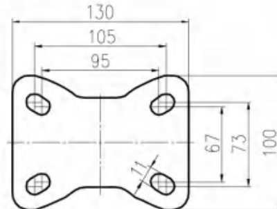
平底固定底板 Plate of Rigid Caster
