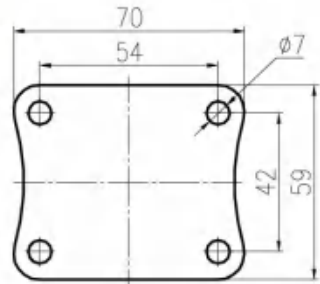
平底活动 刹车底板 Plate of Swivel Caster
