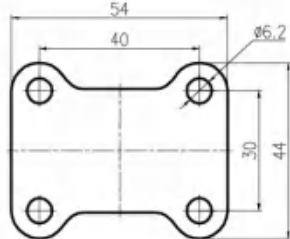
平底固定底板 Plate of Rigid Caster
