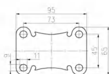
平底固定底板 Plate of Rigid Caster
