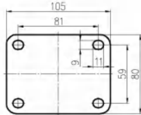
平底活动 刹车底板 Plate of Swivel Caster
