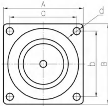
平底活动 刹车底板 Plate of Swivel Caster
