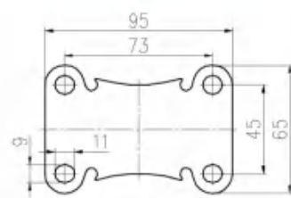
平底固定底板 Plate of Rigid Caster
