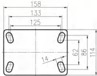
平底活动 刹车 / 固定底板 Plate of Swivel / Rigid Caster
