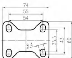
平底固定底板 Plate of Rigid Caster
