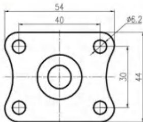
平底活动 刹车底板 Plate of Swivel Caster
