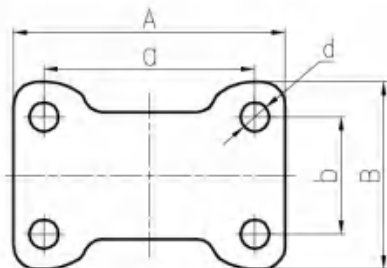
平底固定底板 Plate of Rigid Caster
