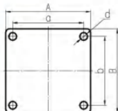
平底活动 刹车底板 Plate of Swivel Caster
