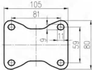
平底固定底板 Plate of Rigid Caster
