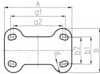
平底固定底板 Plate of Rigid Caster
