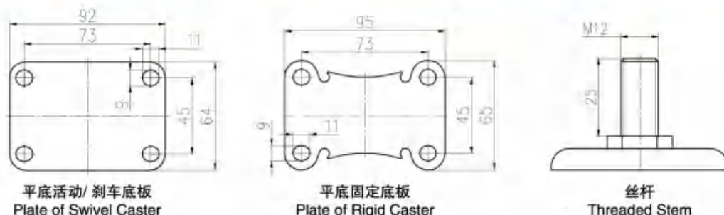
安装尺寸 Installation Drawing
