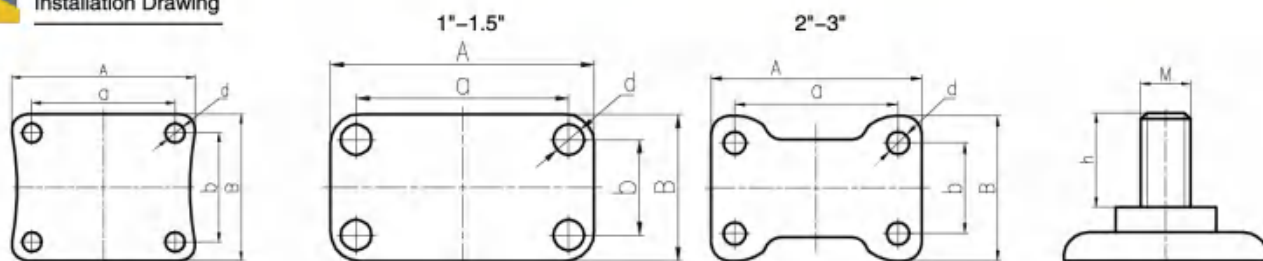
平底活动 刹车底板 Plate of Swivel Caster
