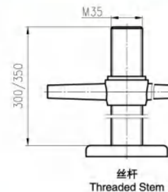
安装尺寸 Installation Drawing
