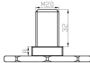
安装尺寸 Installation Drawing
