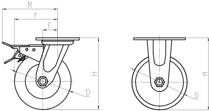
可选拉环刹 Optional Pull Ring Brake
