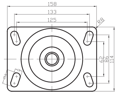
平底活动 刹车 / 固定底板 Plate of Swivel / Rigid Caster
