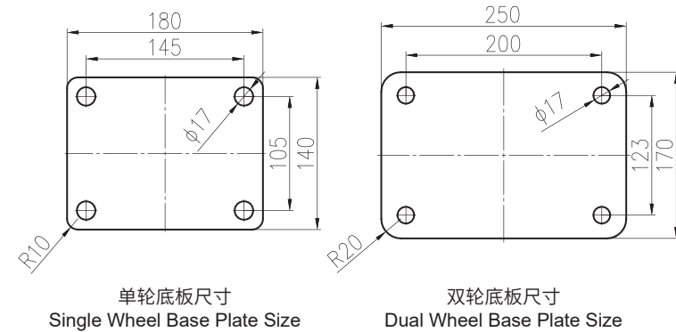
安装尺寸 Installation Drawing
