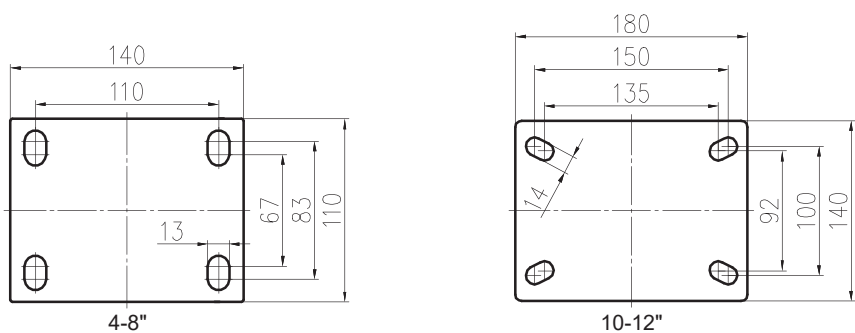
安装尺寸 Installation Drawing
