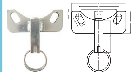
可选拉环刹 Optional Pull Ring Brake
