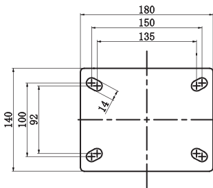
安装尺寸 Installation Drawing
