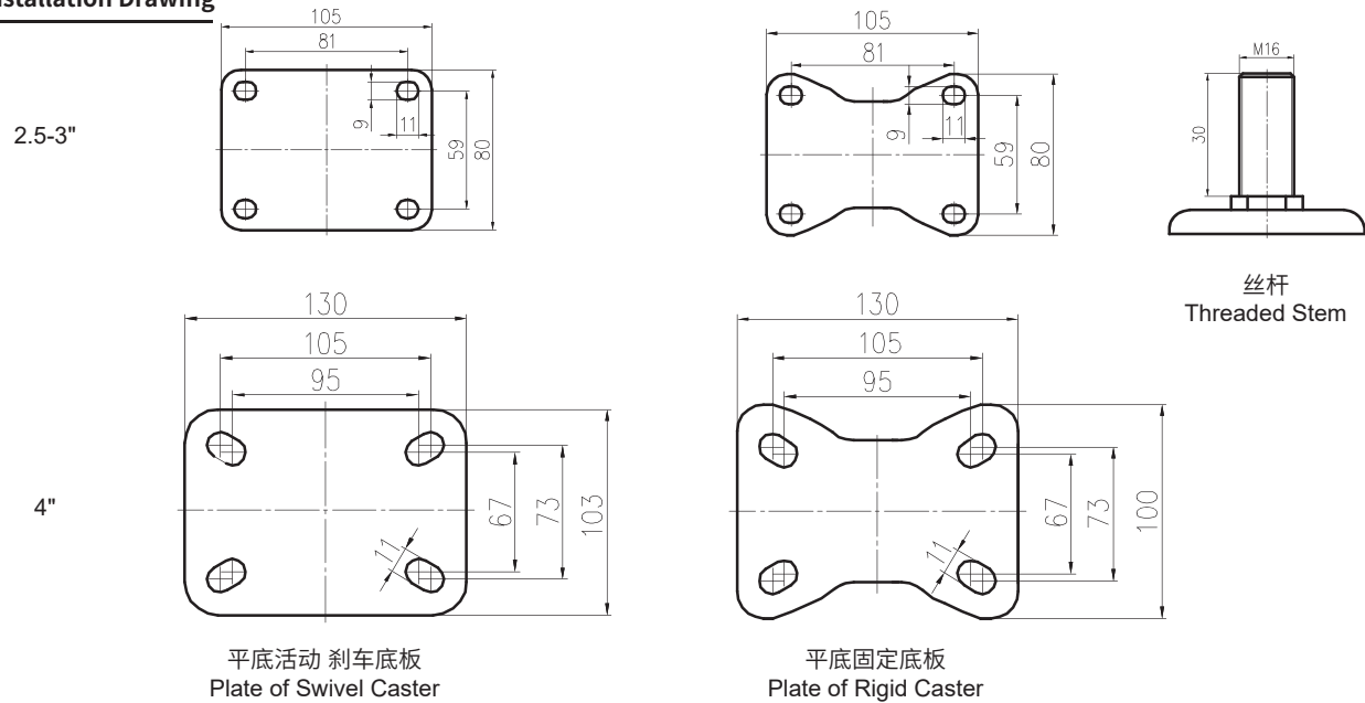
安装尺寸 Installation Drawing
