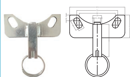
可选拉环刹 Optional Pull Ring Brake
