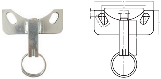
可选拉环刹 Optional Pull Ring Brake
