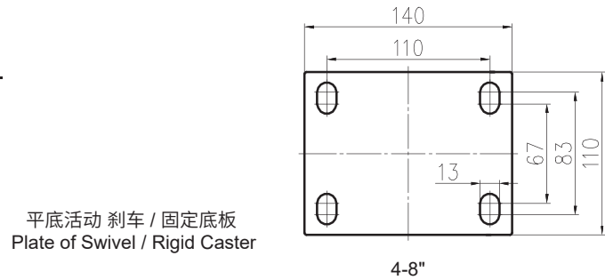
安装尺寸 Installation Drawing
