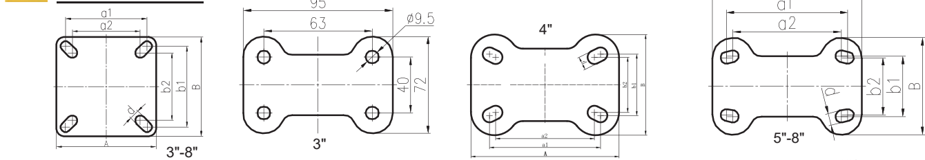
平底活动/ 刹车底板 Plate of Swivel Caster
