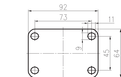
平底活动 刹车底板 Plate of Swivel Caster
