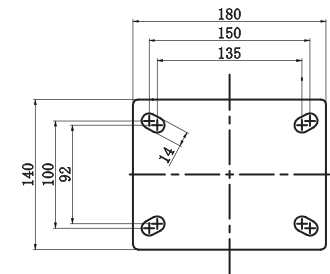
安装尺寸 Installation Drawing
