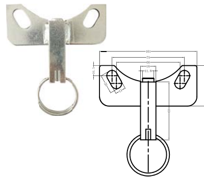
可选拉环刹 Optional Pull Ring Brake
