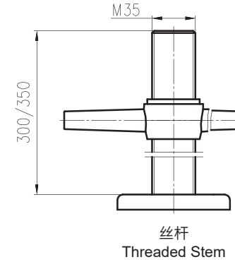
安装尺寸 Installation Drawing
