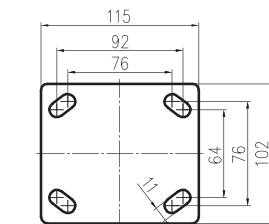
选配底板 Optional Plate
