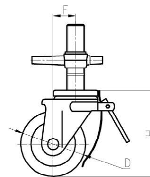
外形尺寸 Overall Dimensions
