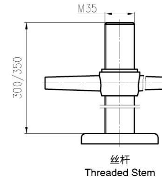
安装尺寸 Installation Drawing
