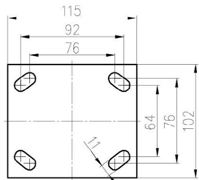
平底活动 刹车 / 固定底板 Plate of Swivel / Rigid Caster
