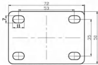
平底活动 刹车底板 Plate of Swivel Caster
