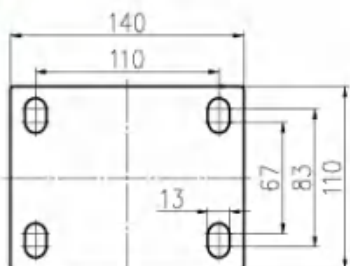
安装尺寸 Installation Drawing
