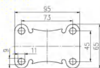
平底固定底板 Plate of Rigid Caster
