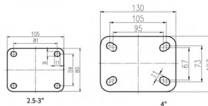
安装尺寸 Installation Drawing
