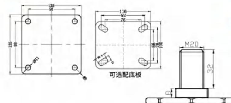
安装尺寸 Installation Drawing
