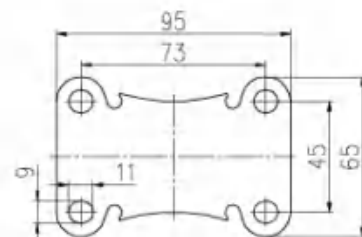
平底固定底板 Plate of Rigid Caster
