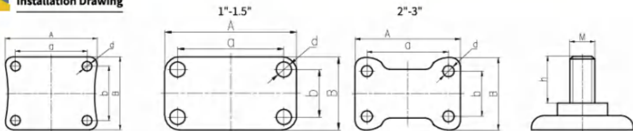
平底活动 刹车底板 Plate of Swivel Caster
