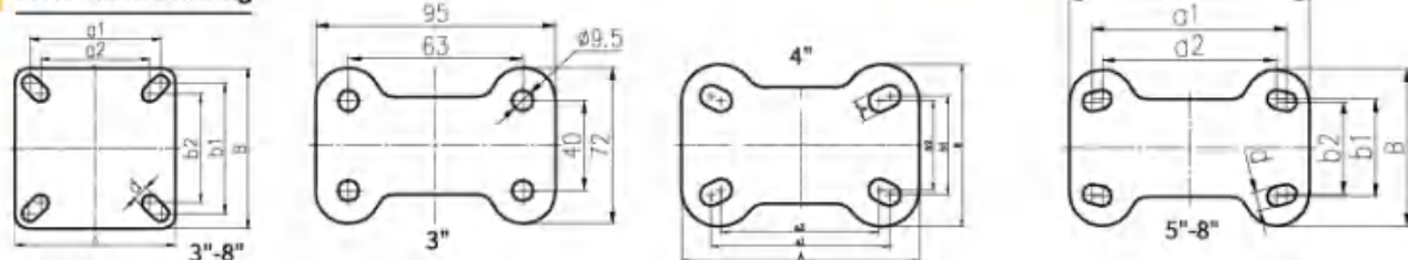
平底活动/ 刹车底板 Plate of Swivel Caster
