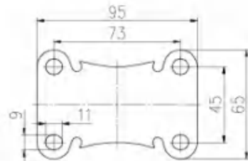
平底固定底板 Plate of Rigid Caster
