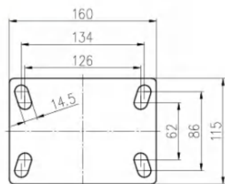
安装尺寸 Installation Drawing
